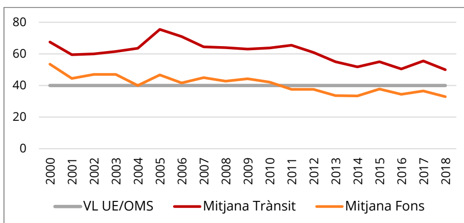
Figura 4. Evolució temporal de la mitjana anual agregada per estacions de trànsit i de fons de NO 2 (en µg/m³) pel període 2000-2018.
