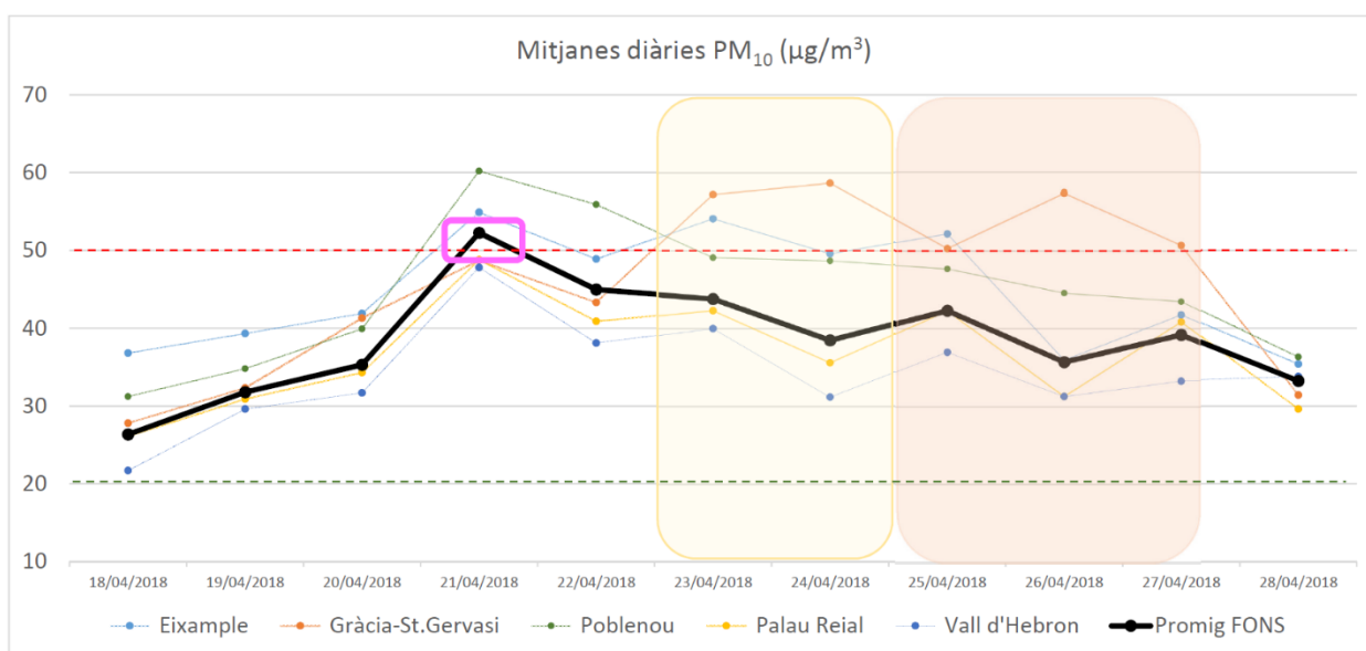
Figura 42. Mitjanes diàries de \text{PM}_{10} ( \mu\text{g}/\text{m}^3 ) a les estacions de la ciutat que mesuren de forma automàtica les partícules \text{PM}_{10} , durant el període analitzat.
