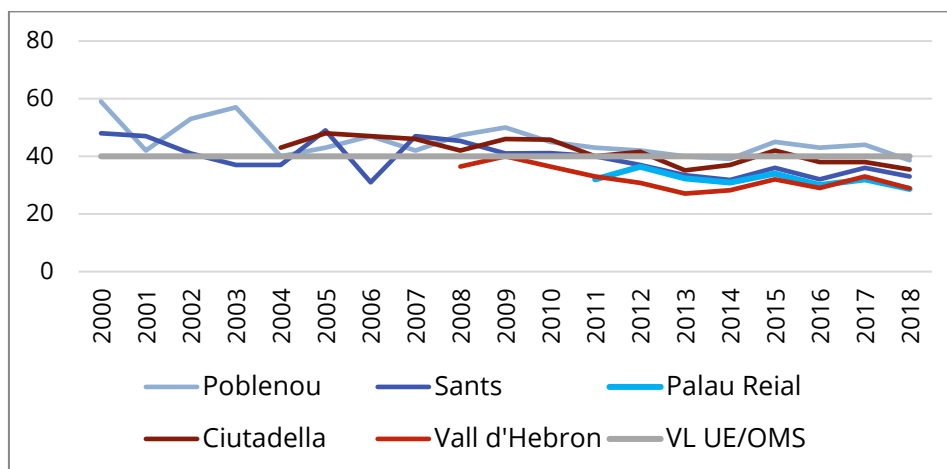
Figura 3. Evolució temporal de la mitjana anual de NO 2 (en µg/m³) pel període 2000-2018 a les estacions de fons de la ciutat.
