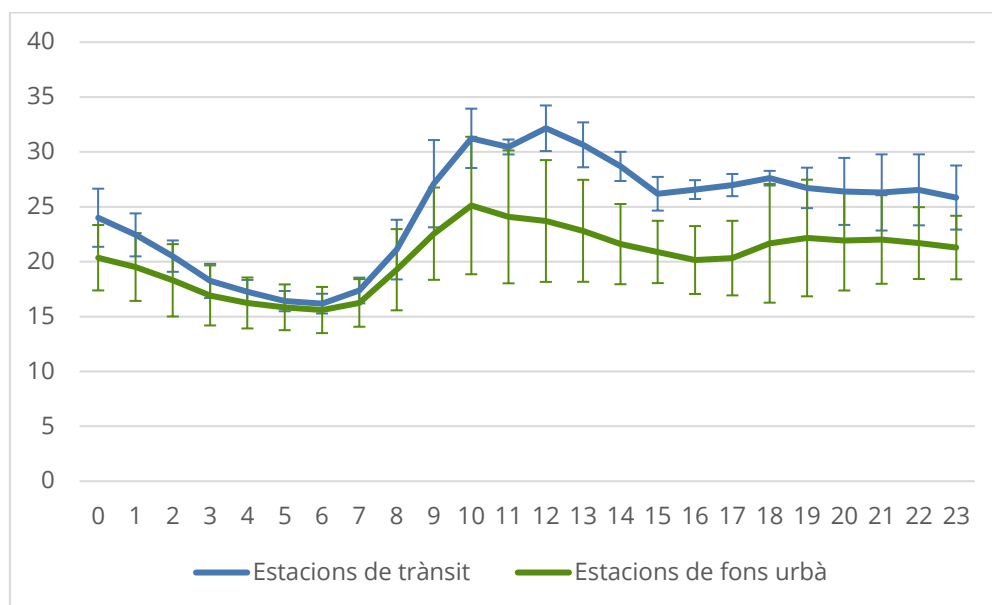
Figura 25. Perfil horari mitjà de PM 10 (mitjana horària en µg/m³) durant el 2018 per a les estacions de trànsit i de fons urbà.
