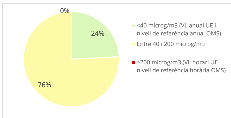
Figura 37. Distribució dels nivells màxims horaris de \text{NO}_2 mesurats a les estacions de la ciutat (en % hores).
