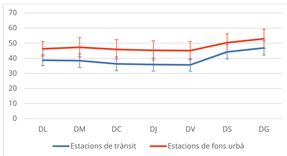
Figura 34. Perfil diari d'O 3 (mitjana diària en µg/m³) durant el 2018 en les estacions de trànsit i de fons urbà.
