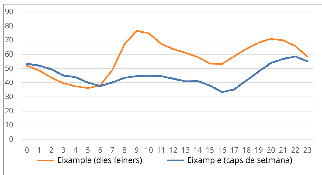
Figura 22. Perfil horari de NO 2 (mitjana horària en µg/m³) durant el 2018 a l'estació de l'Eixample en dies feiners i en caps de setmana.
