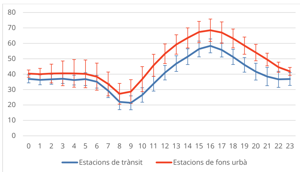
Figura 31. Perfil horari d'O 3 (mitjana horària en µg/m³) durant el 2018 en les estacions de trànsit i de fons urbà.
