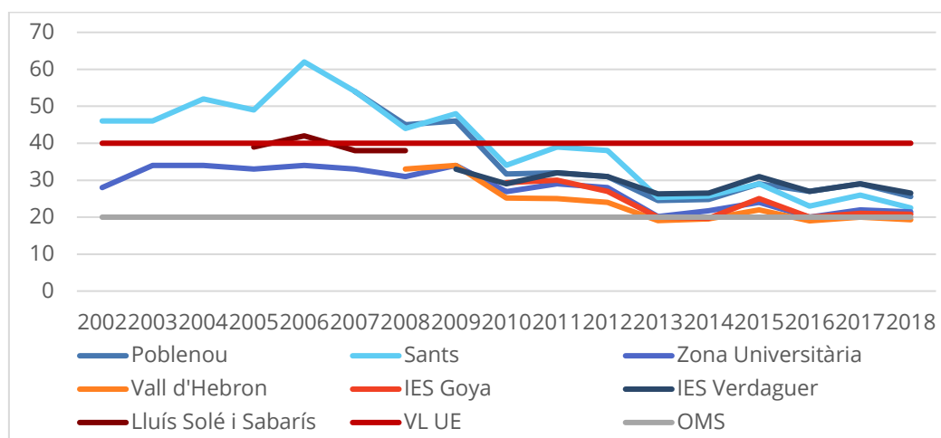
Figura 8. Evolució temporal de la mitjana anual de PM_{10} (en \mu g/m^3 ) pel període 2002-2018 a les estacions de fons urbà.
