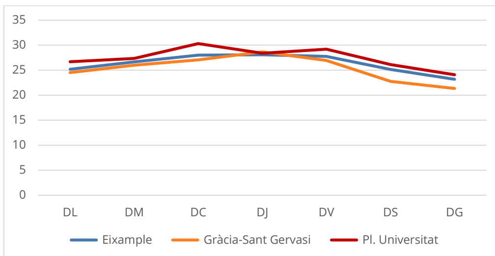
Figura 27. Perfil setmanal de PM 10 (mitjana diària en µg/m³) durant el 2018 en les estacions de trànsit.
