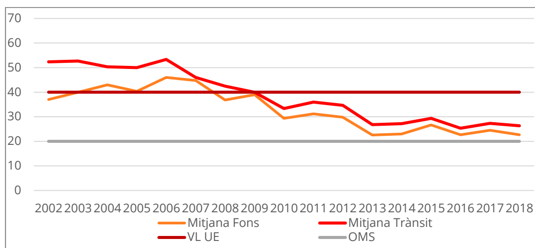
Figura 9. Evolució temporal de la mitjana anual agregada per estacions de trànsit i de fons de PM_{10} (en \mu g/m^3 ) pel període 2002-2018.
