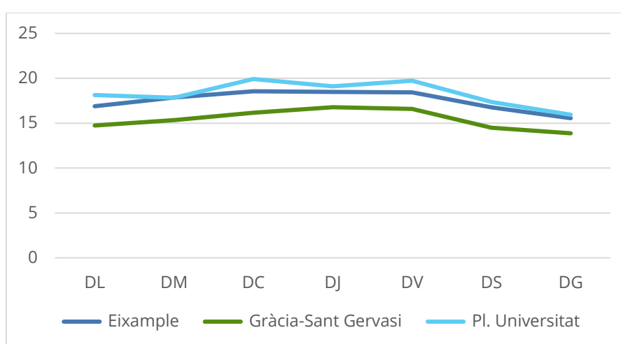
Figura 29. Perfil setmanal de PM 2,5 (mitjana diària en µg/m³) durant el 2018 en les estacions de trànsit.
