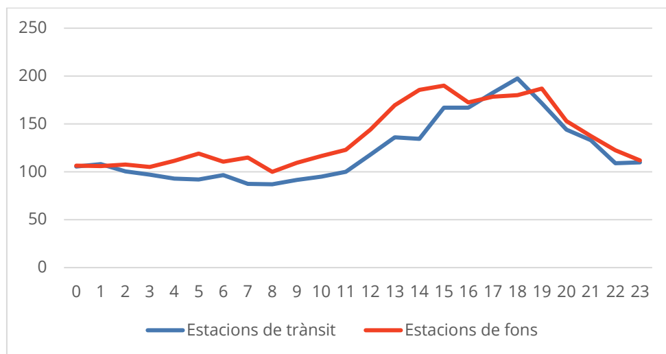
Figura 32. Perfil màxim horari d'O 3 (màxim horari en µg/m³) durant el 2018 en les estacions de trànsit i de fons urbà.
