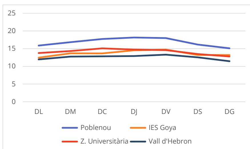
Figura 30. Perfil setmanal de PM 2,5 (mitjana diària en µg/m³) durant el 2018 en les estacions de fons urbà.
