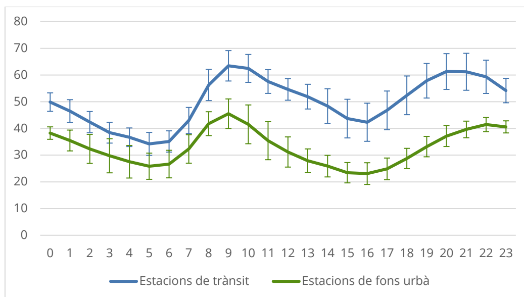
Figura 21. Perfil horari mitjà de NO 2 (mitjana horària en µg/m³) durant el 2018 per a les estacions de trànsit i de fons urbà.
