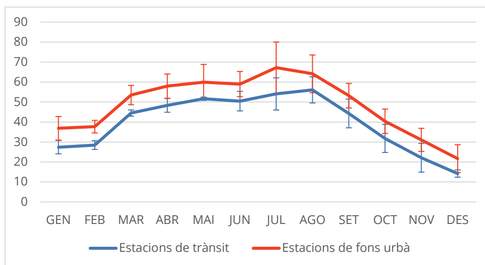
Figura 33. Perfil horari d'O 3 (mitjana horària en µg/m³) durant el 2018 en les estacions de trànsit i de fons urbà.
