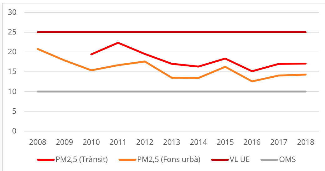
Figura 14. Evolució temporal de la mitjana anual agregada per estacions de trànsit i de fons de PM_{2,5} (en \mu g/m^3 ) pel període 2008-2018.
