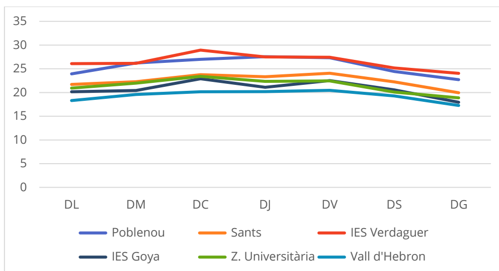
Figura 28. Perfil setmanal de PM 10 (mitjana diària en µg/m³) durant el 2018 en les estacions de fons urbà.
