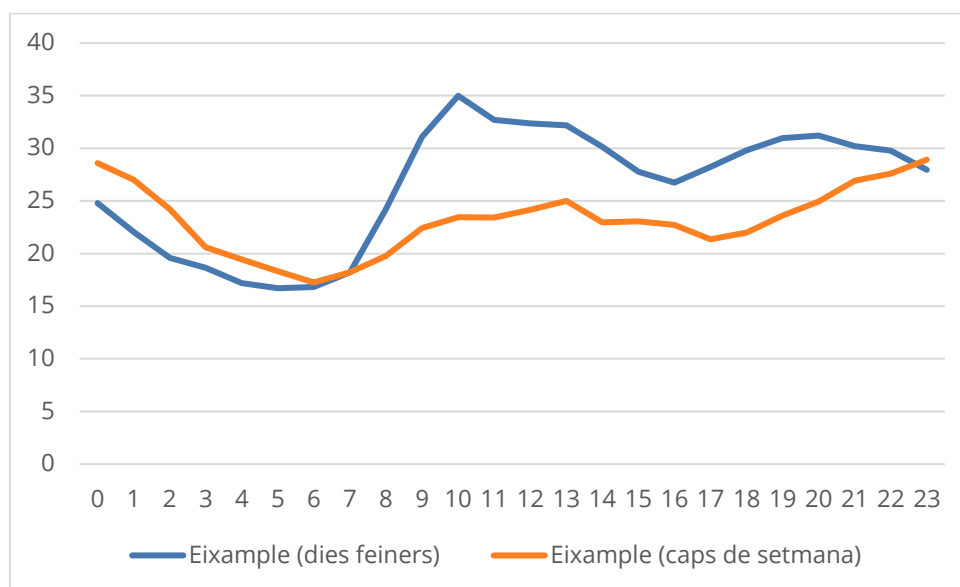
Figura 26. Perfil horari de PM 10 (mitjana horària en µg/m³) durant el 2018 a l'estació de l'Eixample en dies feiners i en caps de setmana (dades del monitor automàtic tipus TEOM).
